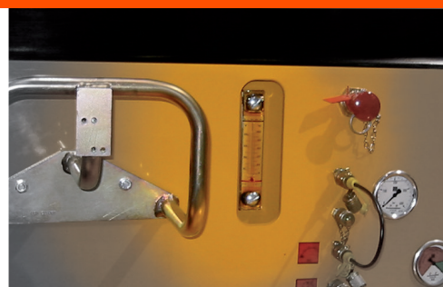
Exemple d'application de l'indicateur de niveau à colonne avec thermomètre HCX
