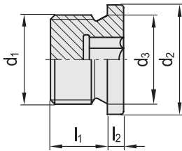
DIN 908-ST-A
