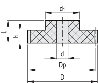
ZCP-2.0 (Z ≤ 16)
