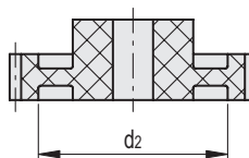
ZCP-1.0 (Z ≥ 17)
