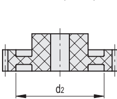
ZCP-2.0 (Z ≥ 17)
