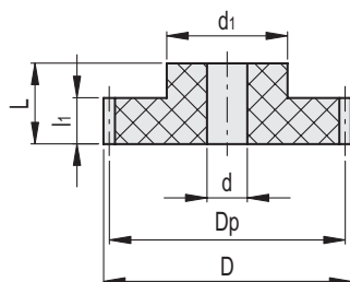
ZCP-1.0 (Z ≤ 16)
