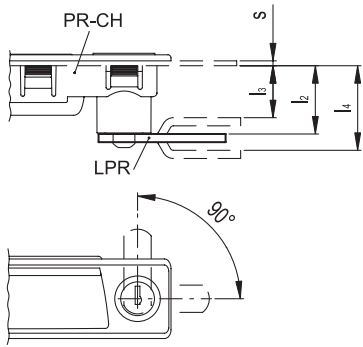
Montaggio su maniglia PR-CH
