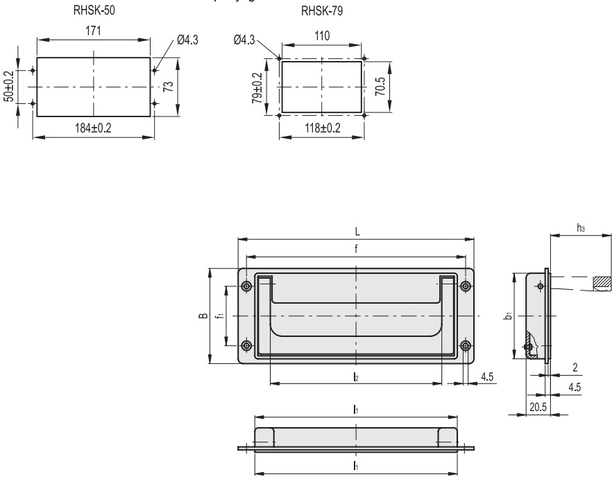
Gabarits de perçage
