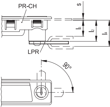
Assemblage sur poignée PR-CH
