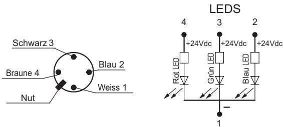
Version mit Kabelstecker
