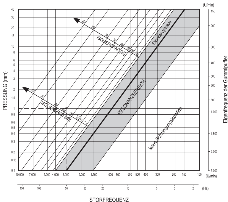
Diagramm zur Überprüfung des Isoliergrades der Gummipuffer
