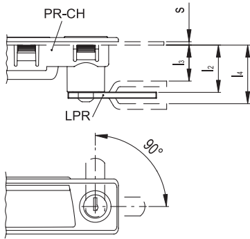
Montage von Griffmulden PR-CH
