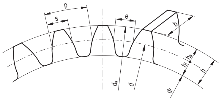
Fig.1: en kuggprofil
